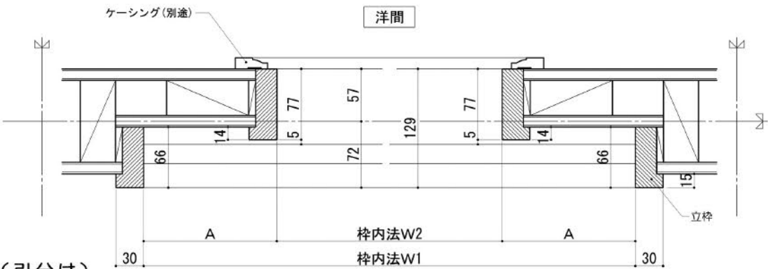
平面図 (引分け)
