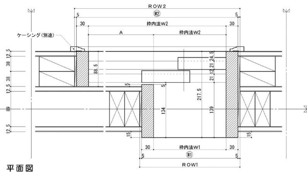
2XNo.28-2620-217 和室～洋間 洋間側2本引込み戸枠
