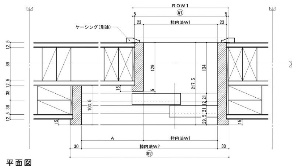
2XNo.27-2620-217 和室～洋間 和室側2本引込み戸枠
