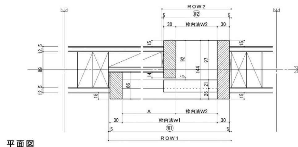
2XNo.13-1720-144 和室～和室(広縁)境 片引き戸枠
